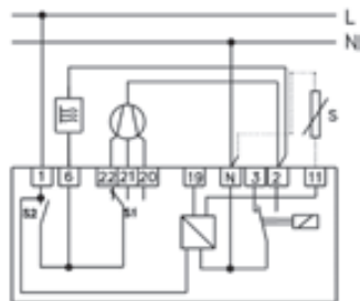
ESQUEMA 9: Fan-coil a dos tubos. Sólo calefacción. Regulación sobre válvula y ventilador.
