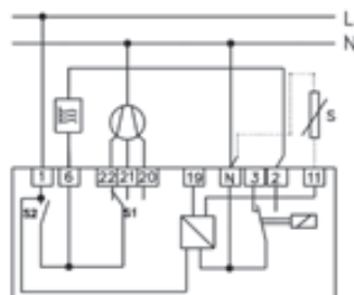
ESQUEMA 7: Fan-coil a dos tubos. Sólo calefacción. Regulación sobre válvula y mando sobre ventilador.
