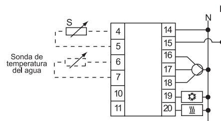
ESQUEMA 3: Fan-coil a cuatro tubos.
