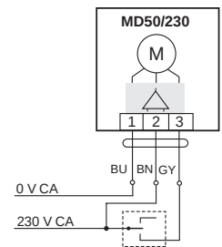
Control a 2 puntos
