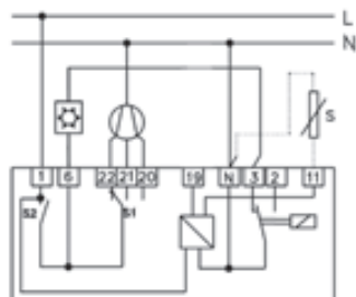
ESQUEMA 6: Fan-coil a dos tubos. Sólo refrigeración. Regulación sobre válvula y mando sobre ventilador.
