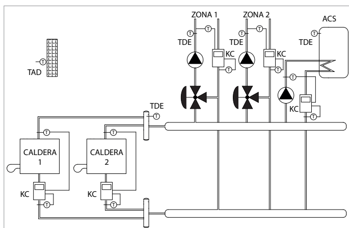
Dos calderas con dos circuitos de calefacción y producción de A.C.S.
