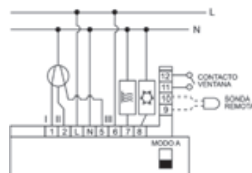
ESQUEMA 2: Fan-coil a cuatro tubos con cambio frío/calor local o Bomba de calor con dos maniobras independientes, una de frío y otra de calor.
