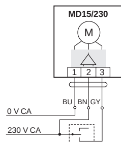
Control a 2 puntos
