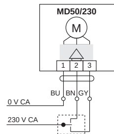
Control a 3 puntos
