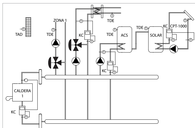
Caldera con un circuito de calefacción, piscina y producción de A.C.S. con calentamiento solar.
