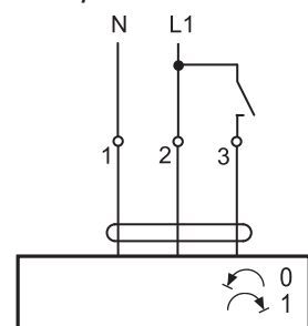
Control todo/nada
