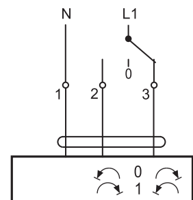
Control a tres puntos
