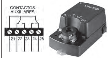
CONTROL TODO/NADA
