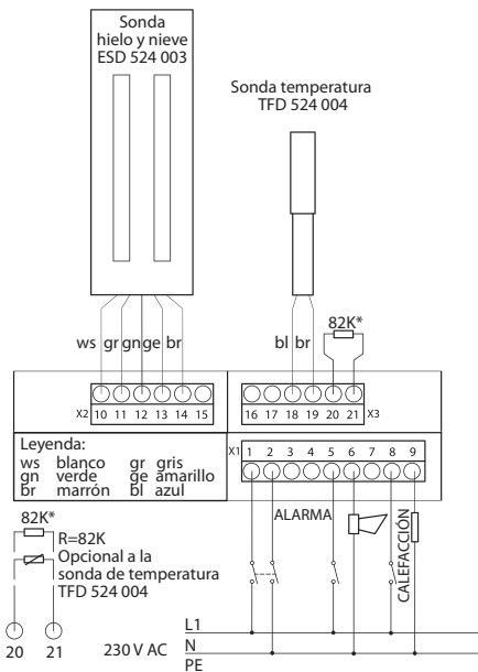
Esquema de conexión de la central de hielo y nieve con las sondas ESD 524 003 y TFD 524 004 para canalones
