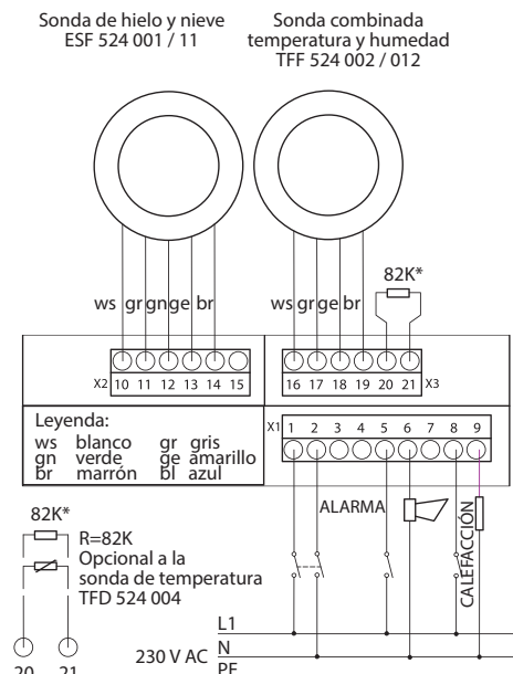
Esquema de conexión de la central de hielo y nieve con las sondas ESF 524 001/011 y TFF 524 002/012 para espacios abiertos
